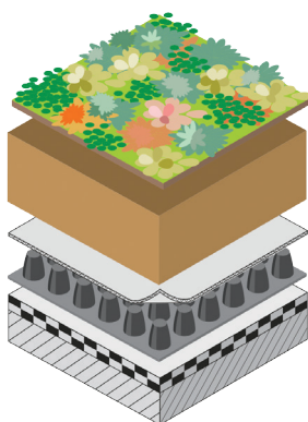
Opbouw Nophadrain Extensief Groendaksysteem
