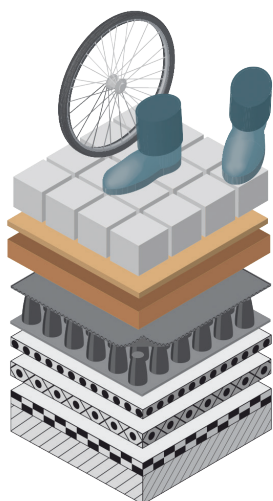
Opbouw Nophadrain Terrasdaksysteem met ND 220 Drainagesysteem
