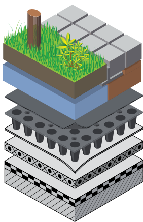
Opbouw Nophadrain Intensief Groendaksysteem
