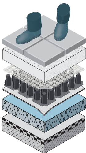
Opbouw met ND TRASDRAIN® 200hsv Drainagesysteem
