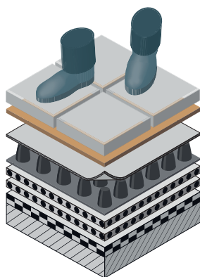
Aufbau Nophadrain Terrassensystem
