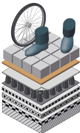
Aufbau Nophadrain Terrassensystem mit ND 220 Drainagesystem
