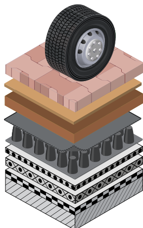
Aufbau Parkdachsystem - Lkw (Belastungsklasse 3) mit ND 600hd
