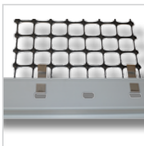
Das ND Steildach Extensiv Erosionsschutzsystem mit ND Erosionsschutzprofil
