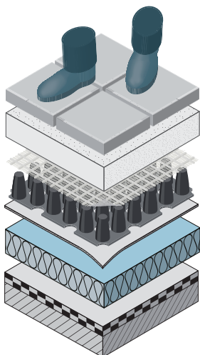
Aufbau mit ND TRASDRAIN® 200hsv Drainagesystem
