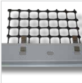
Fixierung von ND ESG-40/40 an ND Erosionsschutzprofil mit ND Befestigungsclips
